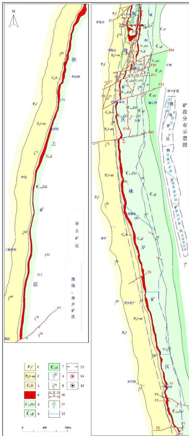
图 3.3.2 燕坨矿床矿区地质图(翁申富等, 2019)
