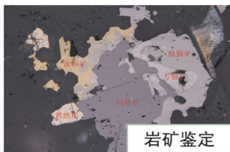
独居石背散射图
