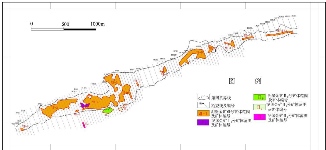
图 3.5.7 泥堡金矿床氧化矿VII及层状矿体 I、II 矿体分布（据贵州省地质矿产勘查开发局一〇五地质大队，2020）
